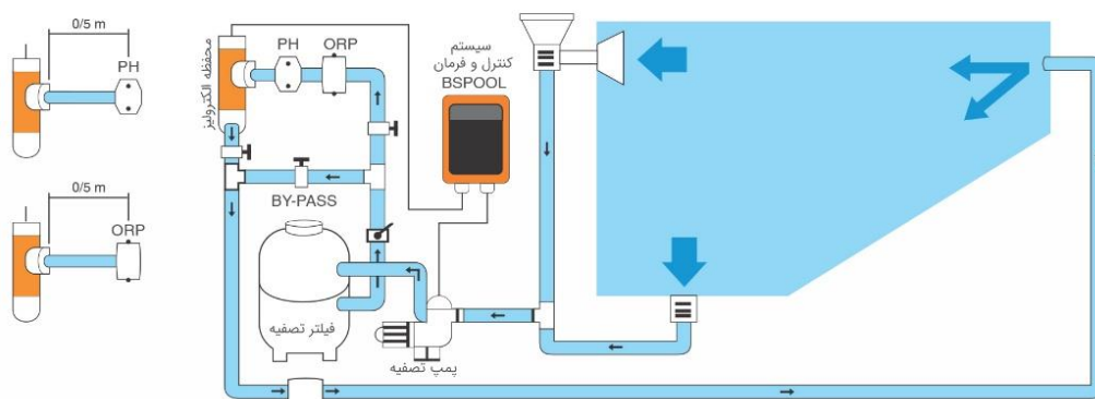
■ نصب کلرزن نمکی در سیستم استخر
